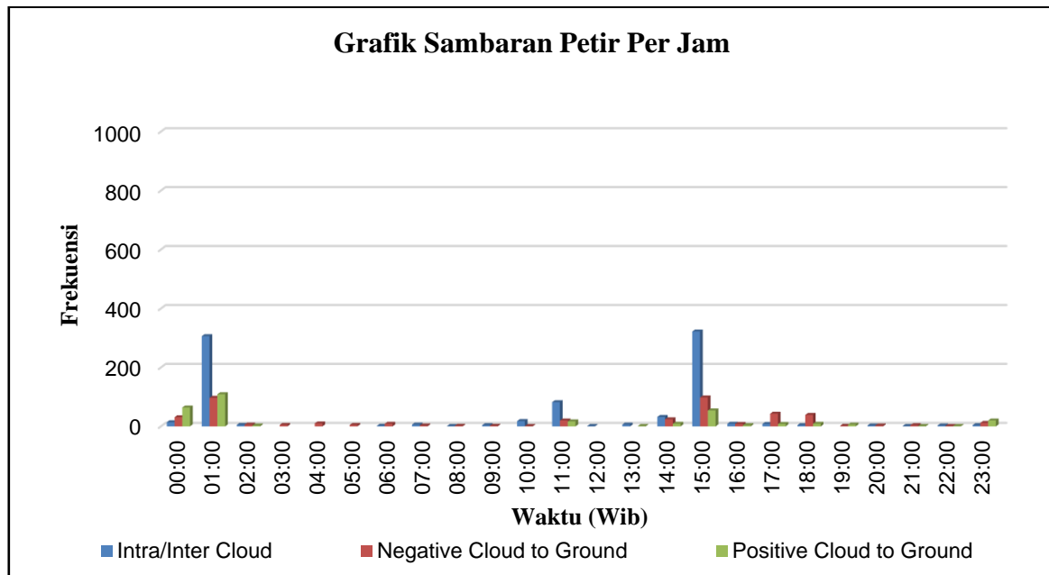
Gambar 8. Grafik Jumlah Sambaran Petir Per Jam
