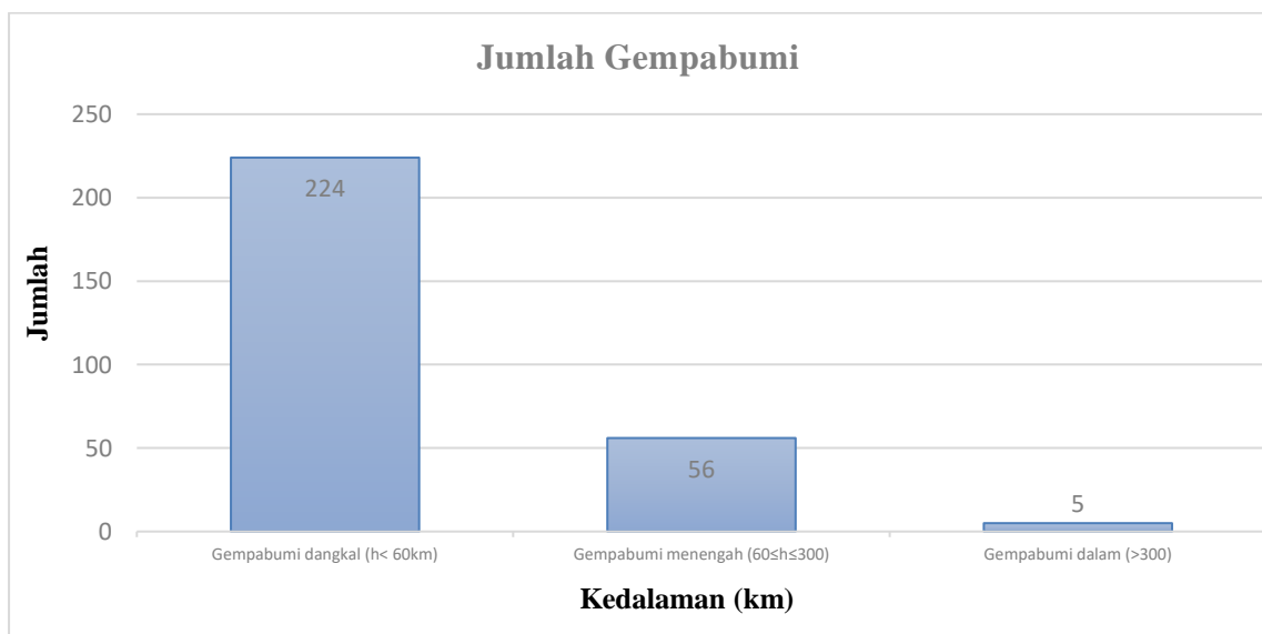
Gambar 3. Jumlah Gempabumi Berdasarkan Kedalaman Hiposenter
