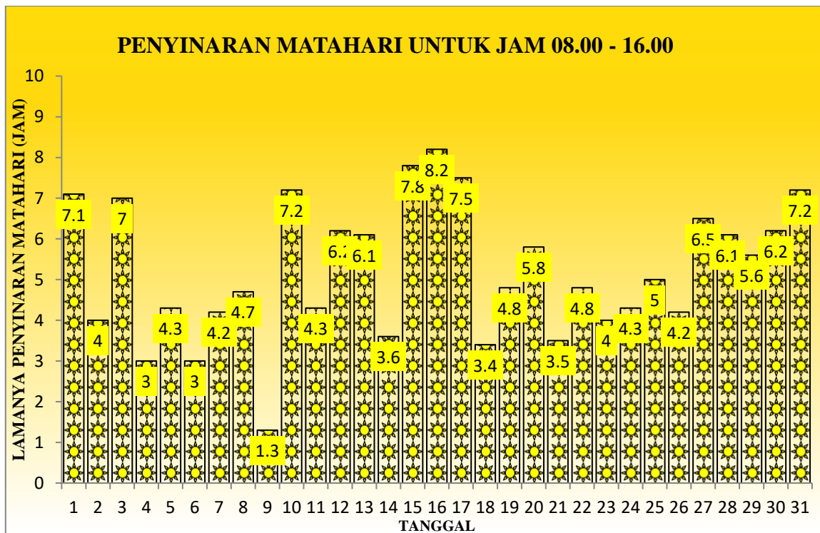
Gambar 15. Grafik Lama Penyinaran Matahari
