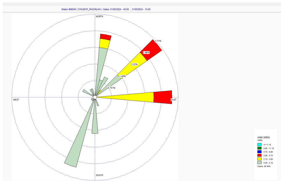
Gambar 14. Grafik Wind Rose
