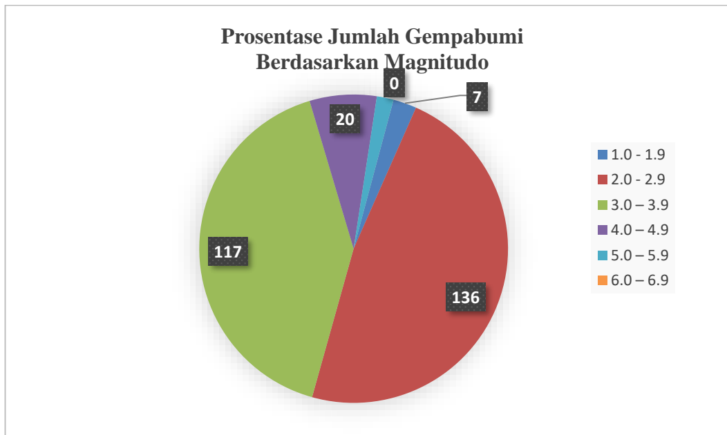
Gambar 2. Frekuensi Gempabumi Berdasarkan Magnitudo
