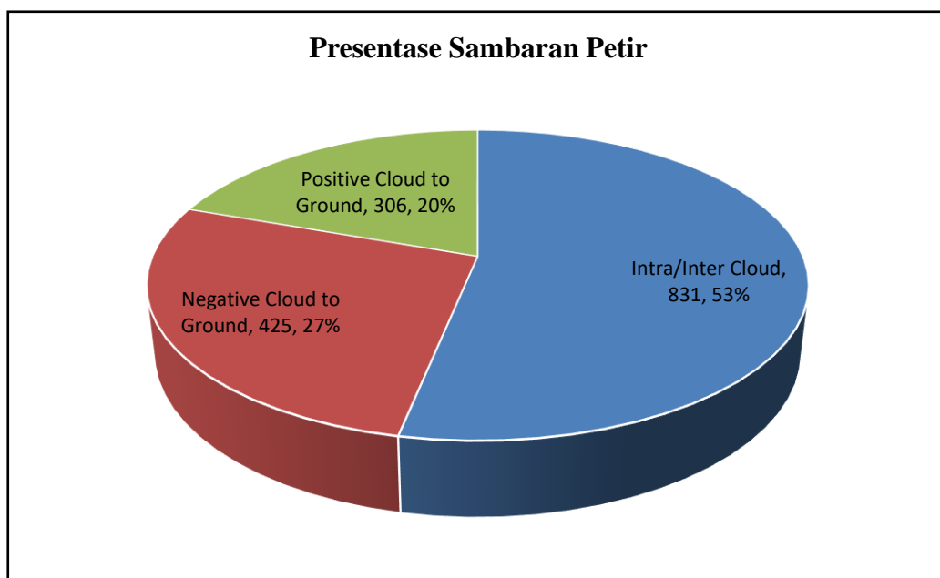
Gambar 5. Total Sambaran Menurut Jenis Muatan
