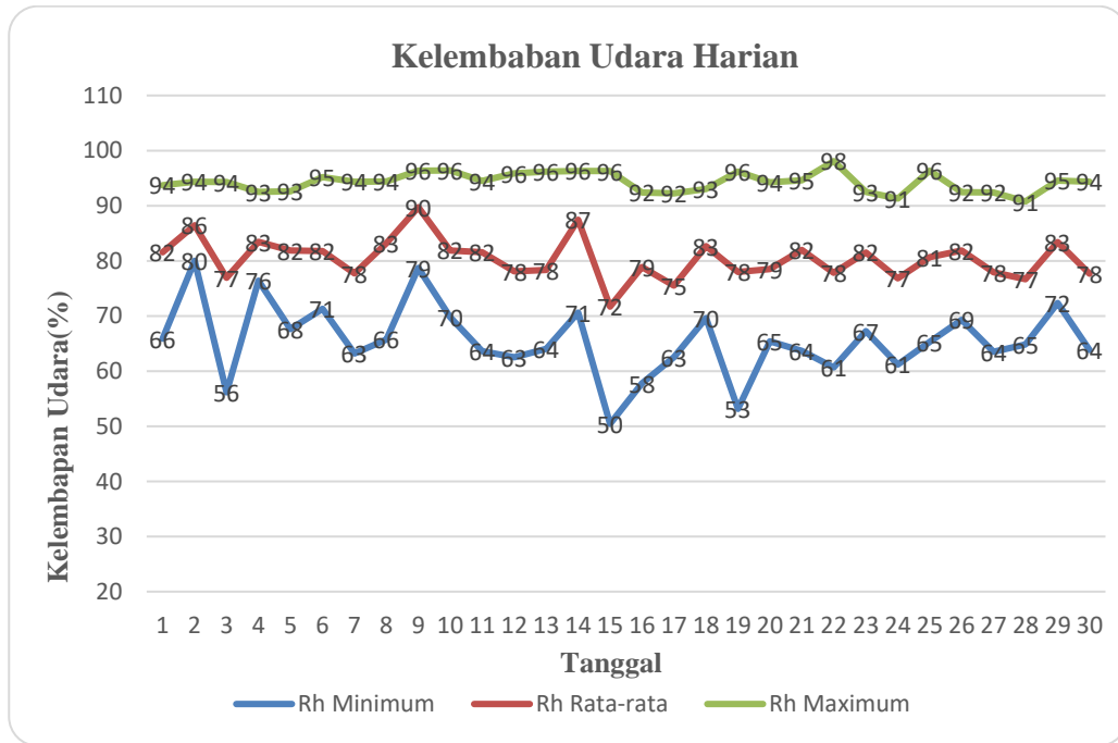
Gambar 13. Grafik Kelembapan Udara Harian
