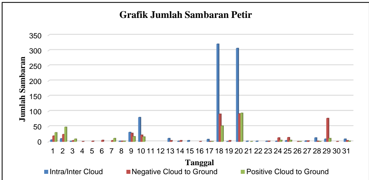
Gambar 6. Jumlah Sambaran Petir
